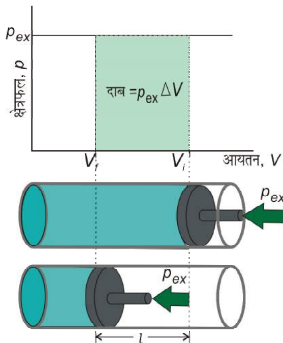
चित्र 6.5 (क) सिलिंडर में स्थित आदर्श गैस पर एक पद में स्थिर बाह्य दाब P_{ex} द्वारा किया गया संकुचन कार्य छायादार क्षेत्र द्वारा दर्शाया गया है।
