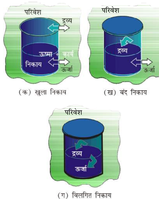
चित्र 6.2 : खुला, बंद एवं विलगित निकाय
